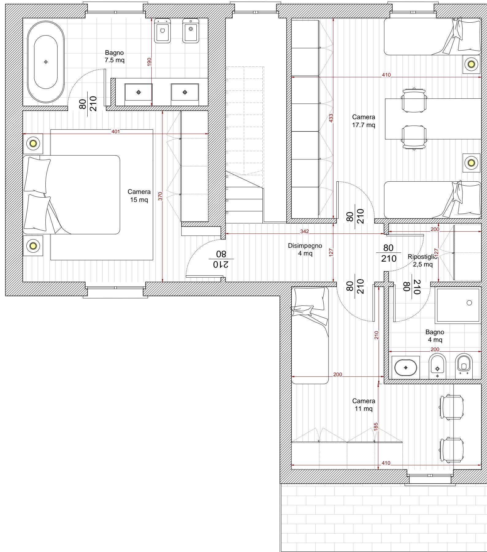
PIANTA PIANO PRIMO - Opzione C
