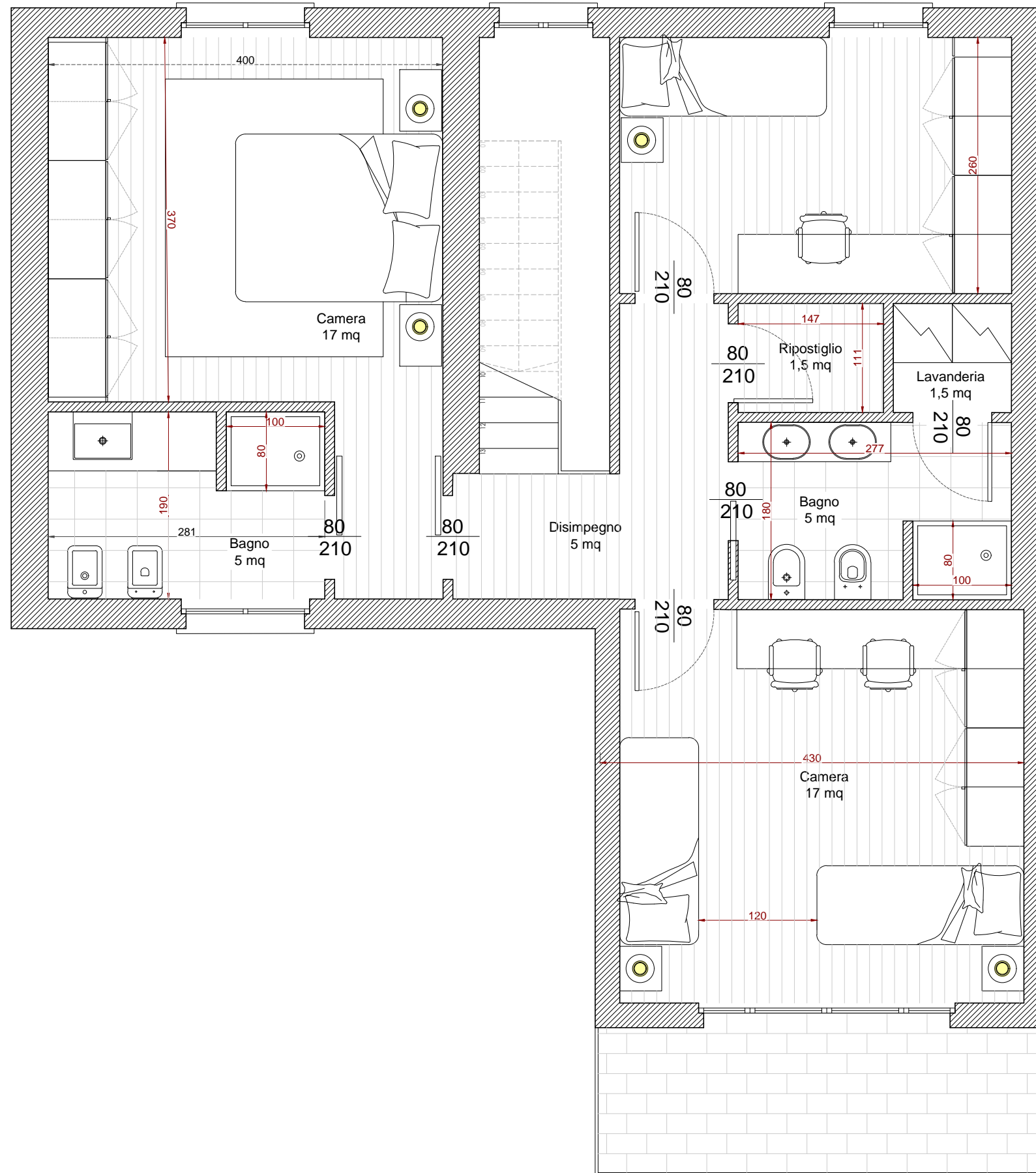
PIANTA PIANO PRIMO - Opzione B
